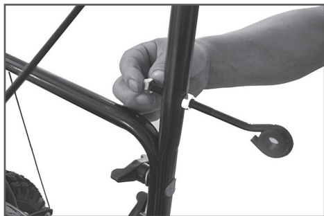
Рис. 13 Монтаж кронштейна рычага поворота желоба
